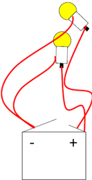
Circuit en dérivation
